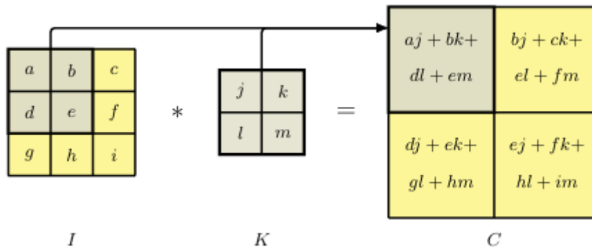
Figura 5: Representação visual da operação de convolução, onde a feature map C é obtida aplicando o filtro K à imagem I
